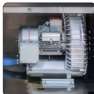
SOUFFLEUR AIR DRY 380 PRO (DE SÉRIE)
